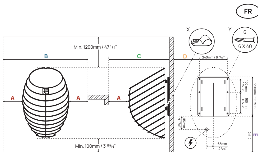
Figure 1. Positionnement du chauffe-sauna.
