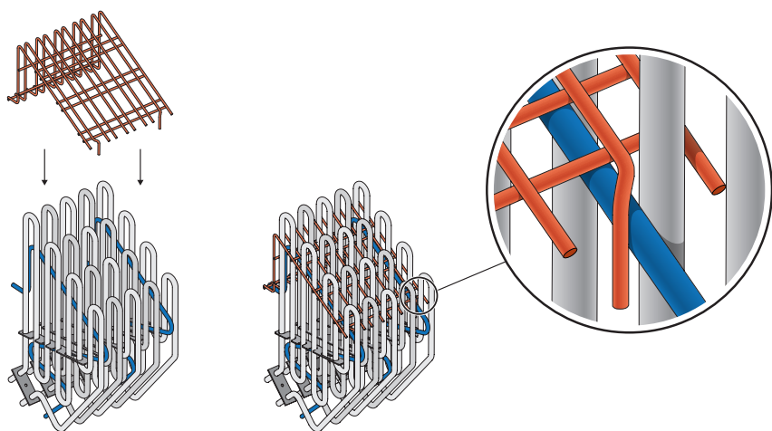
Figure 5. Installation du dispositif de retenue de HUUM DROP 7 et de DROP 9 avec 5 éléments chauffants.
