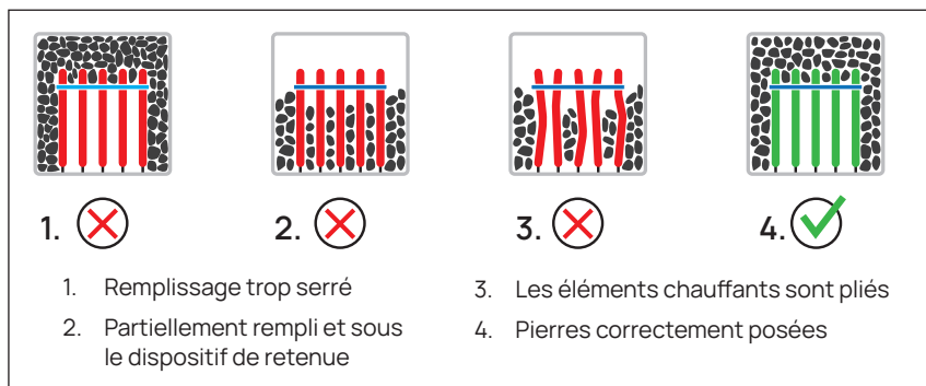
Figure 8. Placez les pierres dans DROP 7 et DROP 9 avec 5 éléments chauffants.
