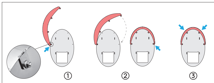
Figure 2. Installation du déflecteur de chaleur.
