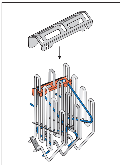
Figure 3. Installation du dispositif de retenue pour HUUM DROP 4 et 6 avec 3 éléments chauffants.
