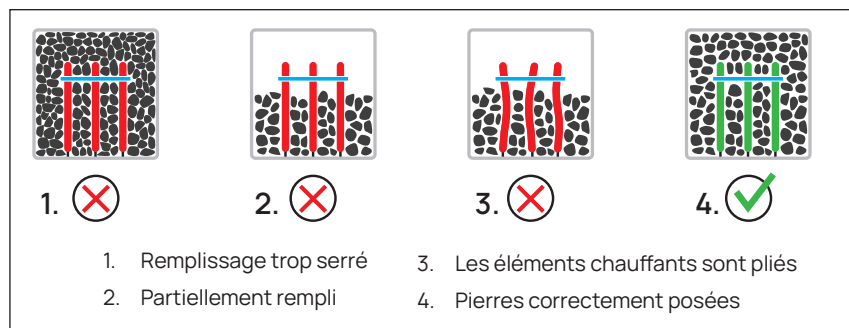
Figure 7. Placez les pierres dans DROP 4 et DROP 6 avec 3 éléments chauffants.
