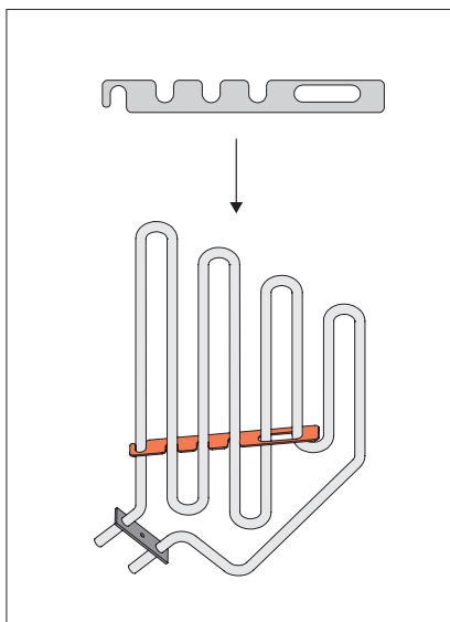
Figure 4. Installation de l'entretoise des éléments chauffants de HUUM DROP.
