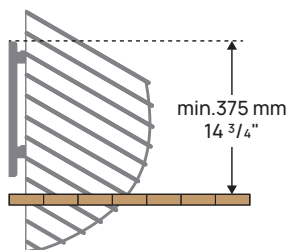
Figure 6. Installation du chauffe-sauna électrique HUUM DROP à l'intérieur du banc de sauna
